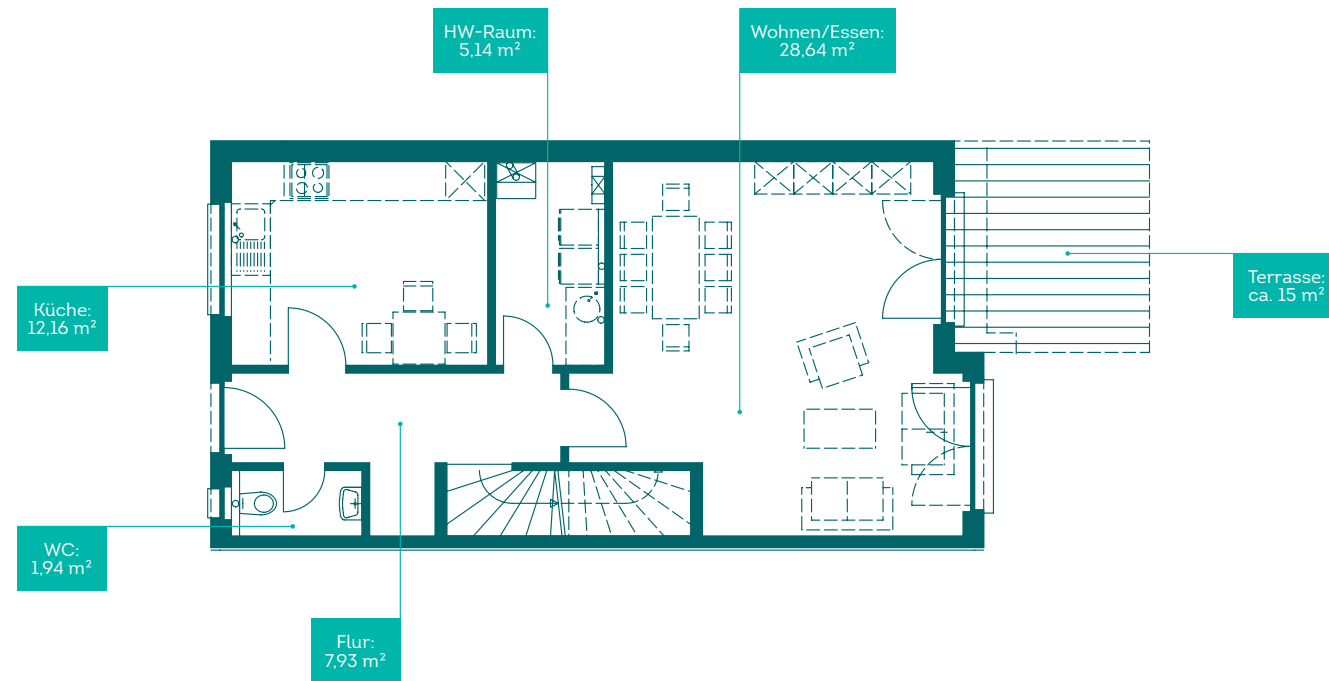
ERDGESCHOSS
