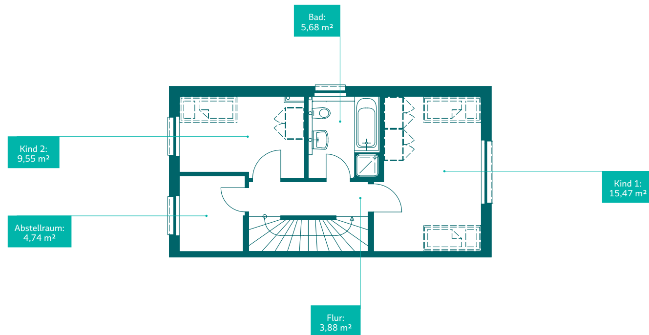
OBERGESCHOSS
